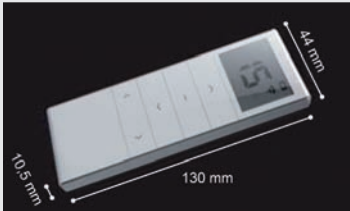
MANDO A DISTANCIA LED 15 CANALES
