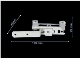
Maestra con Pata
