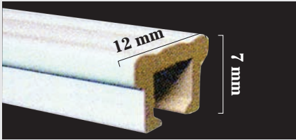
RIEL ALUMINIO A-1
