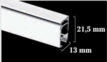
PERFIL RIEL CUBA
