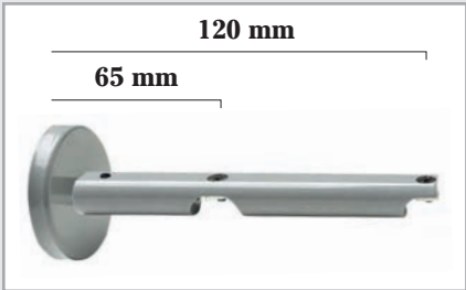
SOPORTE DOBLE FRENTE DECORATIVO
