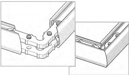
RIEL CON SOPORTE FRENTE DECORATIVO CON VUELTA + CODO Sumar al precio del riel cortado y montado el número de soportes de frente + los codos que necesitamos.
