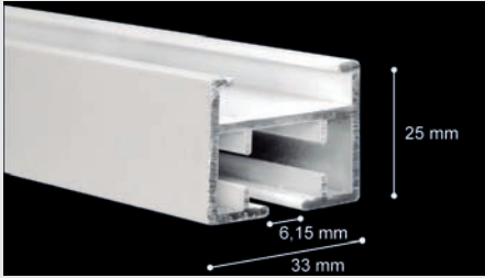
Perfil Riel Motorizado
